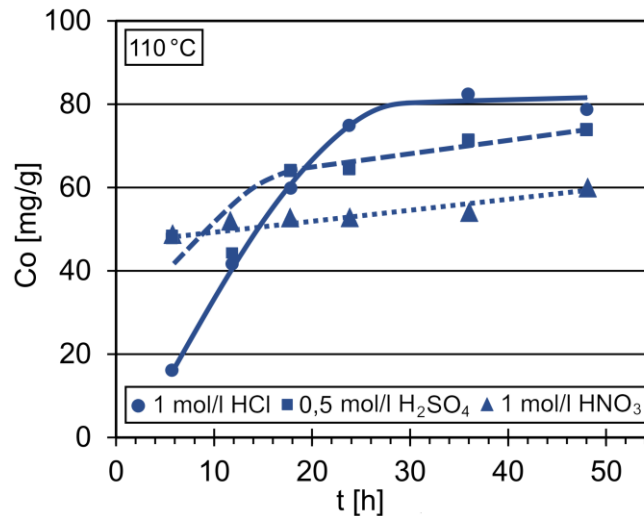
Abbildung 3.6: Gegenüberstellung der Co-Laugung aus einem Hartmetall mittels verschiedener Säuren nach Kojima [8]
