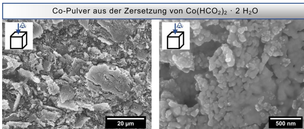
Abbildung 5.36: REM-SE-Aufnahmen des aus der Zersetzung im Rohrofen entstandenen Co-Pulvers
