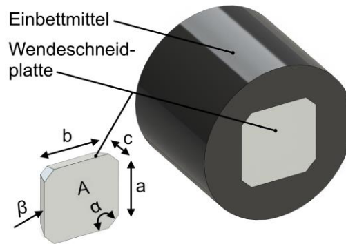
Abbildung 5.17: Geometrie mit Spezifikation des Cermets (links) und Modell des fertigen Probenkörpers für die Tastversuche (rechts)
