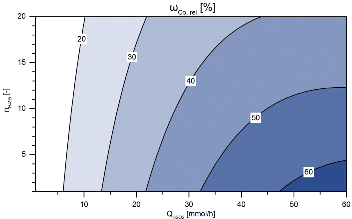
Abbildung 5.28: Konturdiagramm zum Fortschritt der Laugung in 3,75 mol/l CH_2O_2 in Abhängigkeit von den analysierten Faktoren n_{H495} sowie Q_{H2O2}
