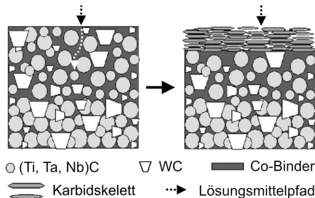
Abbildung 4.4: Korrosionsvorgang nach Barbatti et al. [12]
