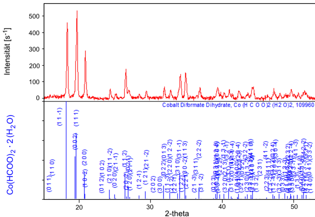
Abbildung 14.2: Röntgendiffraktogramm des Cobaltformiats ( \text{Co}(\text{HCOO})_2 \cdot 2\text{H}_2\text{O} ) aus der vollständigen Laugung mit \text{CH}_2\text{O}_2 + \text{H}_2\text{O}_2 nach 27 d, Kapitel 5.7.2
