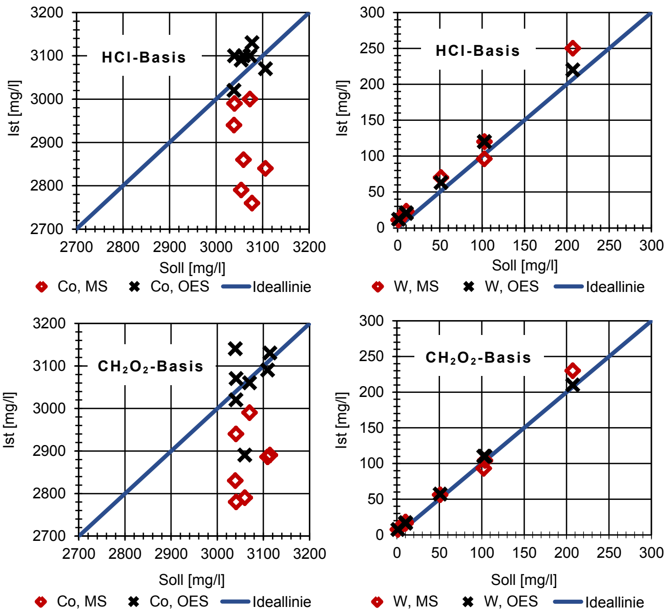
Abbildung 5.22: Analyse der synthetischen Lösungen in HCl sowie CH 2 O 2 jeweils mit H 2 O 2 mittels ICP-MS und -OES
