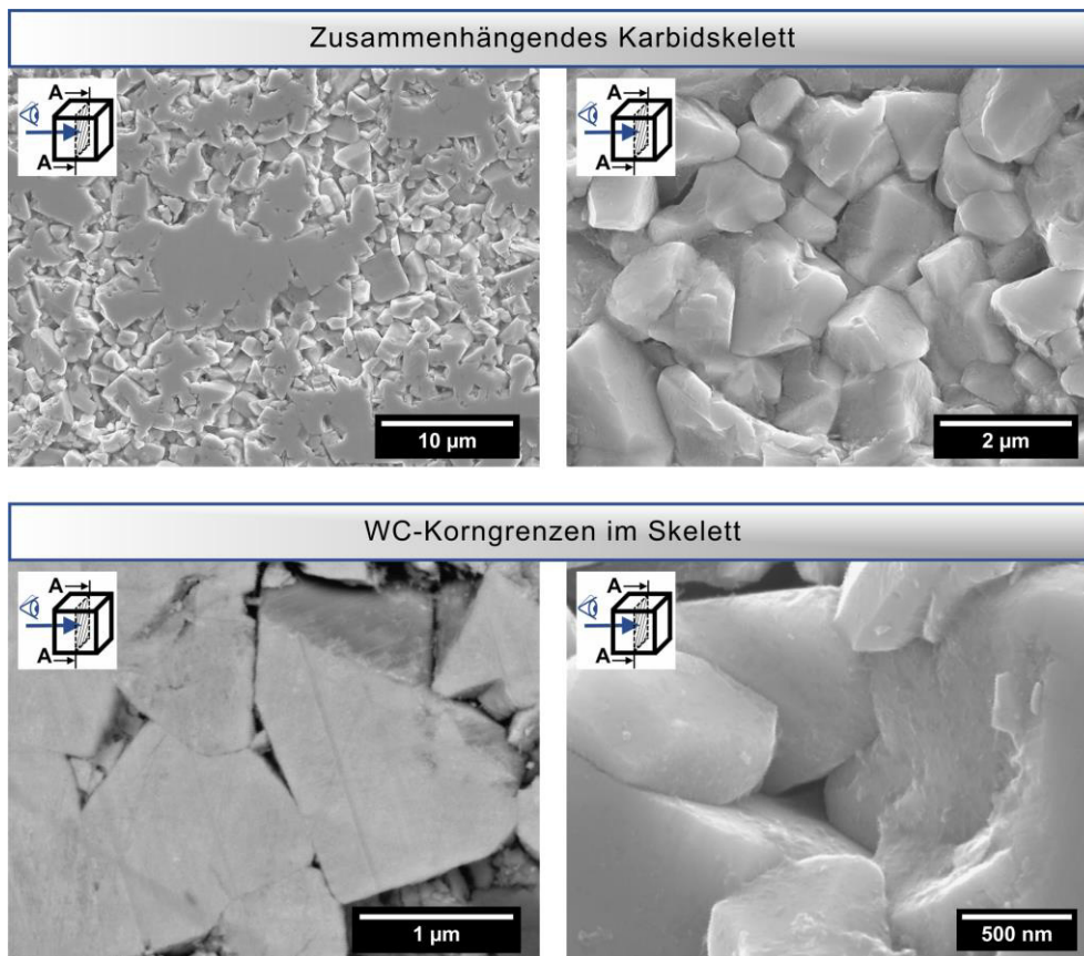
Abbildung 14.3: REM-SE-Aufnahmen des Karbidskeletts aus der vollständigen Laugung in \text{CH}_2\text{O}_2 (Kerne nach Zerkleinerung in der Kugelmühle) mit Details zu den WC-Korngrenzen, Kapitel 5.7.2
