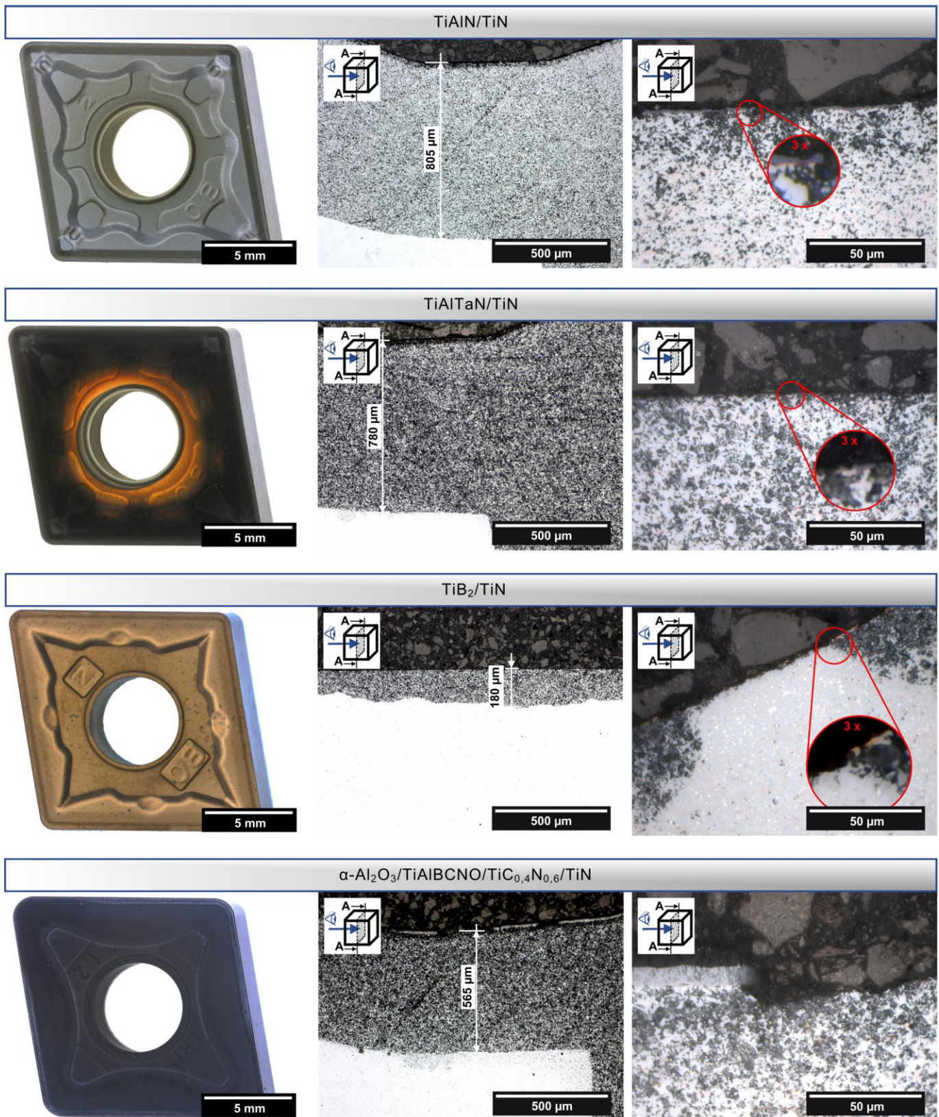
Abbildung 14.4: Resultate der Tastversuche für beschichtete Substrate in 2,0 mol/l HCl bei Q_{\text{H}_2\text{O}_2} = 3,5 \text{ mmol/h} , t = 4 \text{ d} sowie T = 80 \text{ }^\circ\text{C} , Gesamtdarstellung der gelaugten WSP (links), Laugungstiefe im Querschnitt (mittig) und Detail der Beschichtungsreste (rechts) im Lichtmikroskop, Kapitel 5.8
