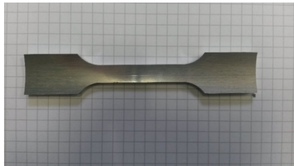
Fig. 9: Tensile specimen
