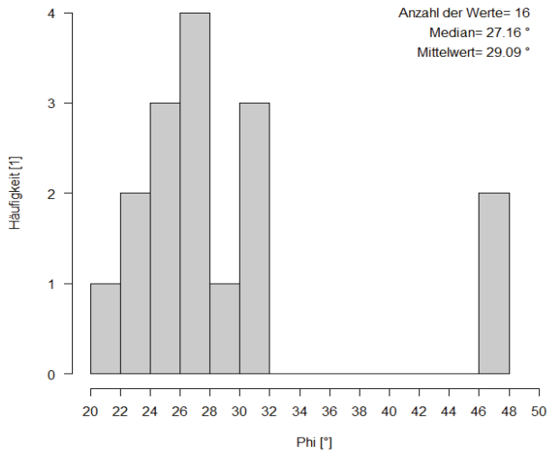
Reibungswinkel
