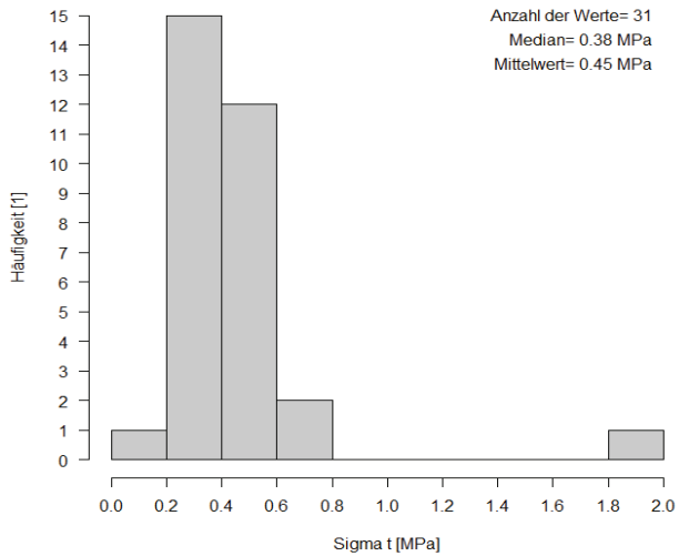
SPZ für tonreiches Haselgebirge
