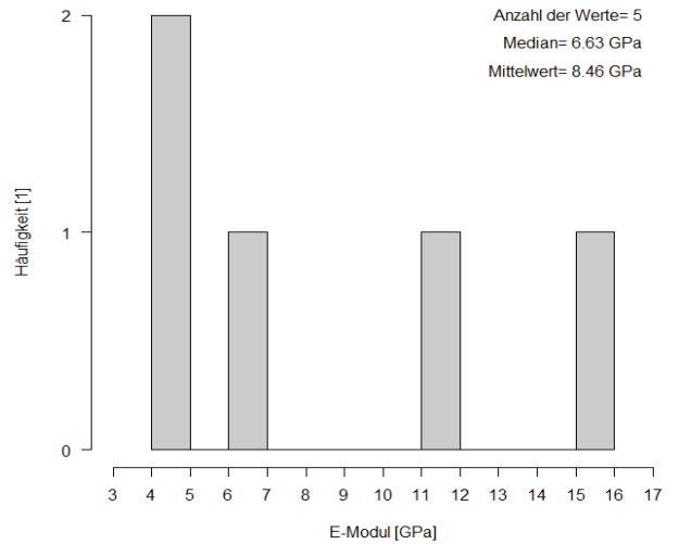
Elastizitätsmodul für tonreiches Haselgebirge
