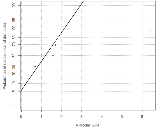
Verformungsmodul für tonreiches Haselgebirge
