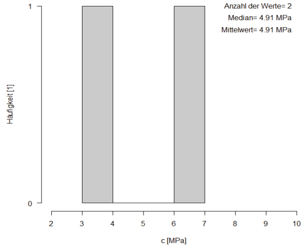
Kohäsion für gipsreiches Haselgebirge
