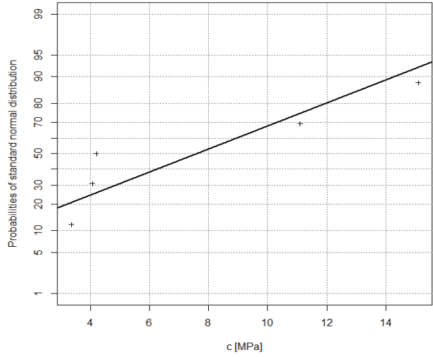
Kohäsion für Dolomit
