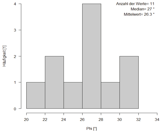
Reibungswinkel für Haselgebirge
