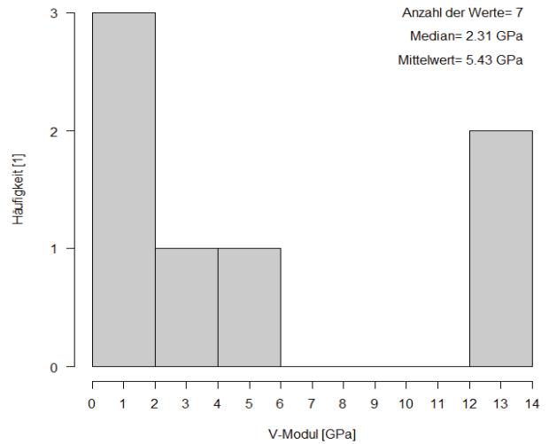
Verformungsmodul gesamt für gipsreiches Haselgebirge
