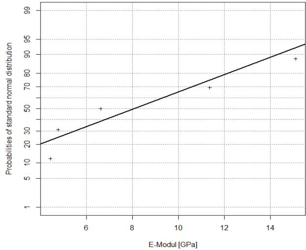
Elastizitätsmodul für tonreiches Haselgebirge
