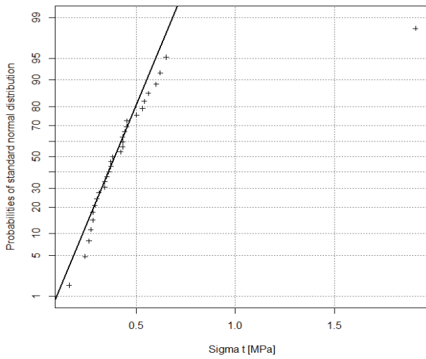
SPZ für tonreiches Haselgebirge
