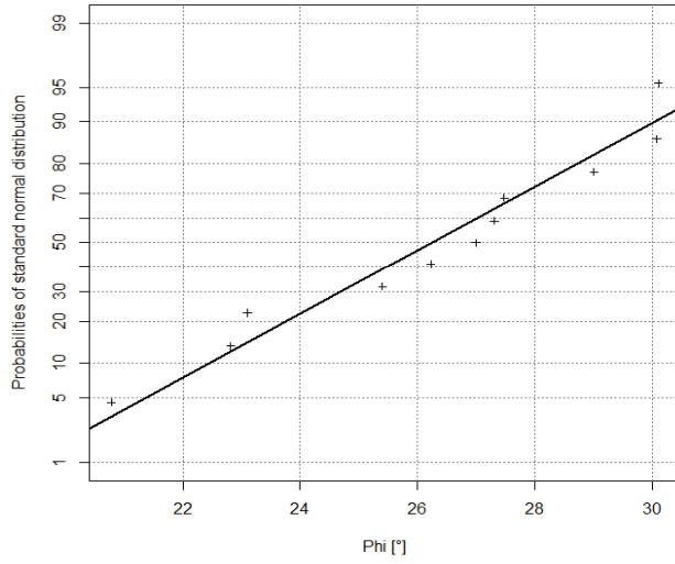
Reibungswinkel für Haselgebirge
