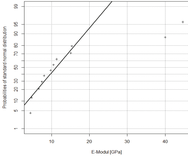
Elastizitätsmodul für Haselgebirge
