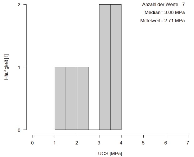
Einaxiale Druckfestigkeit für tonreiches Haselgebirge
