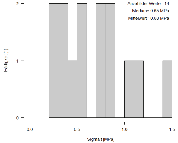
SPZ für gipsreiches Haselgebirge
