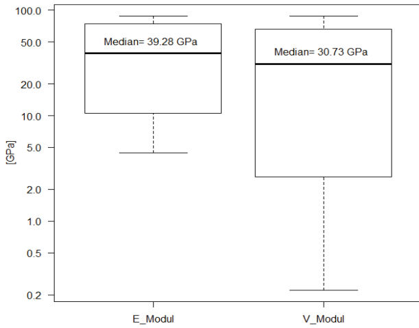
Elastizitäts- und Verformungsmodul
