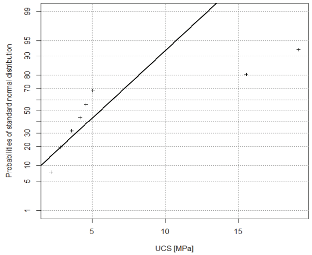
Einaxiale Druckfestigkeit für gipsreiches Haselgebirge
