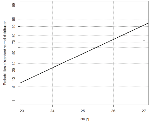
Reibungswinkel für gipsreiches Haselgebirge
