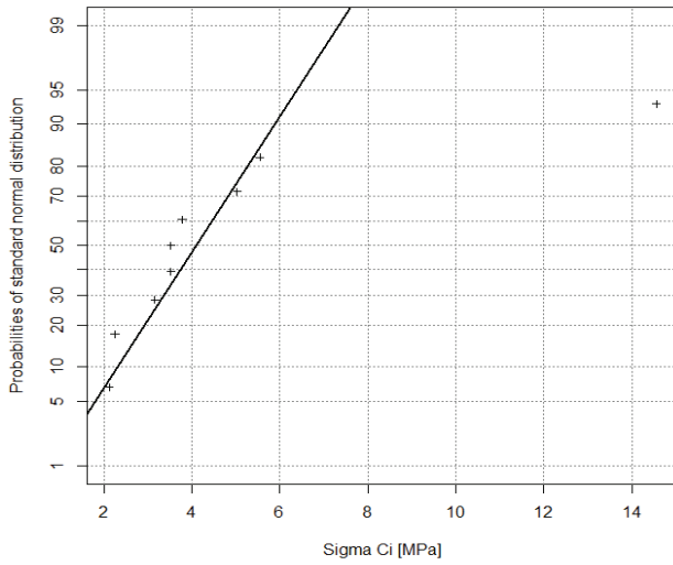
Sigma Ci für tonreiches Haselgebirge
