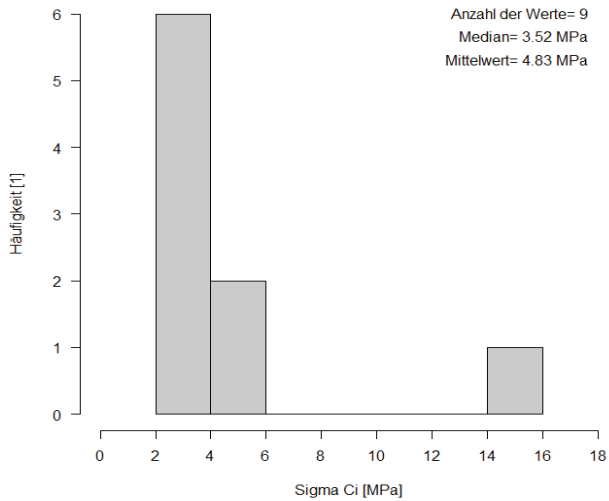
Sigma Ci für tonreiches Haselgebirge
