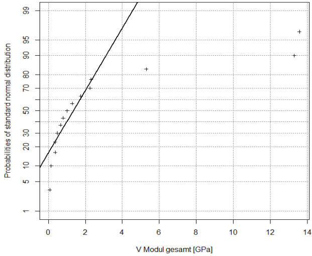
Verformungsmodul gesamt für Haselgebirge
