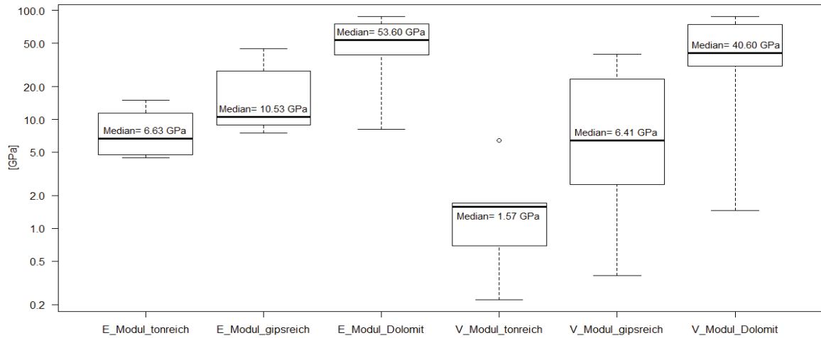
E-Modul und V-Modul für ton-, gipsreiches Haselgebirge und Dolomit
