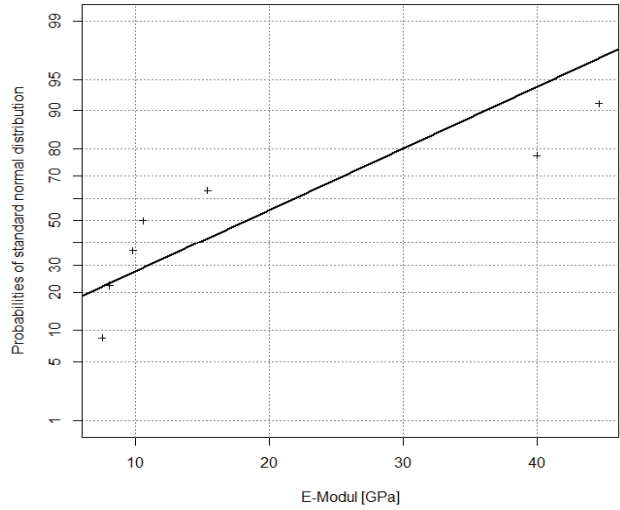
Elastizitätsmodul für gipsreiches Haselgebirge
