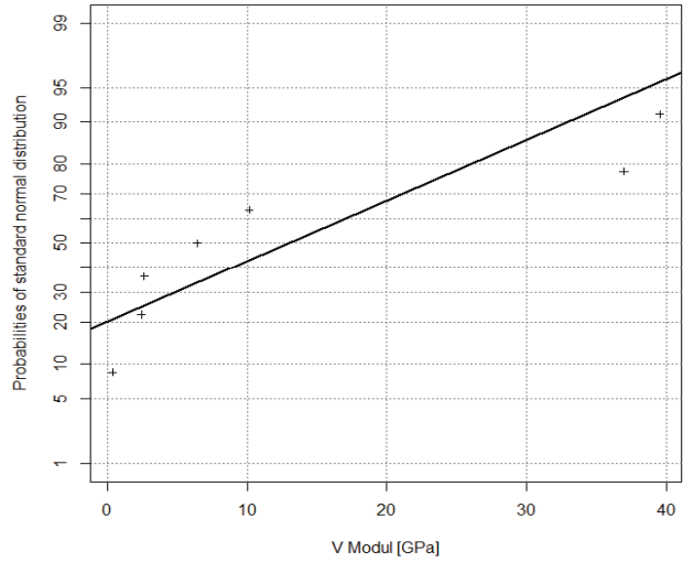
Verformungsmodul für gipsreiches Haselgebirge
