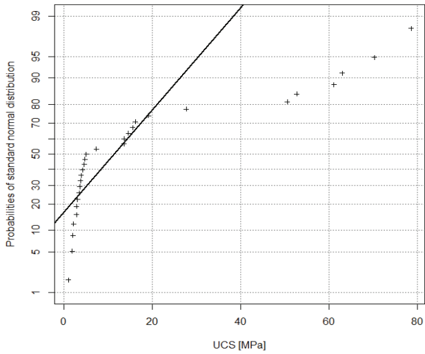
Einaxiale Druckfestigkeit
