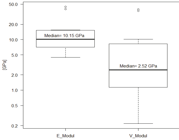
Elastizitäts- und Verformungsmodul für Haselgebirge
