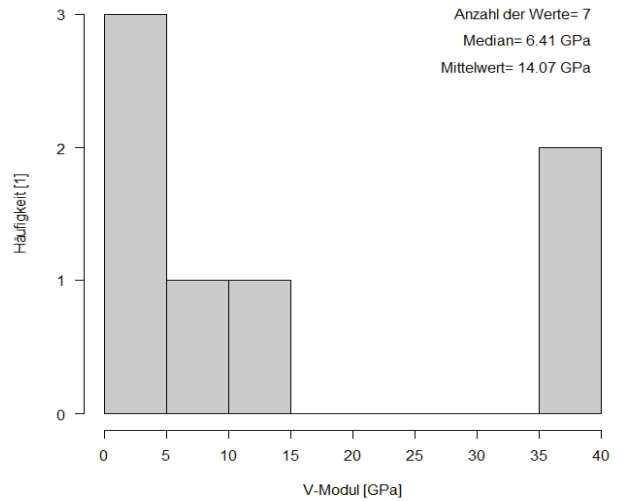
Verformungsmodul für gipsreiches Haselgebirge
