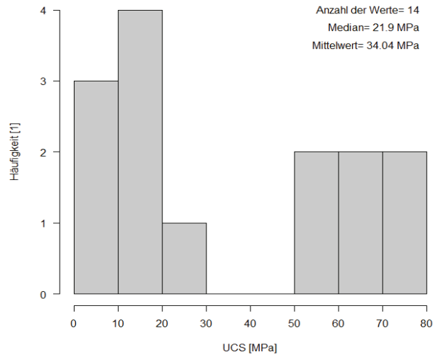
Einaxiale Druckfestigkeit für Dolomit
