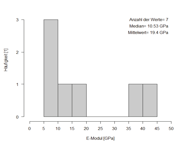
Elastizitätsmodul für gipsreiches Haselgebirge
