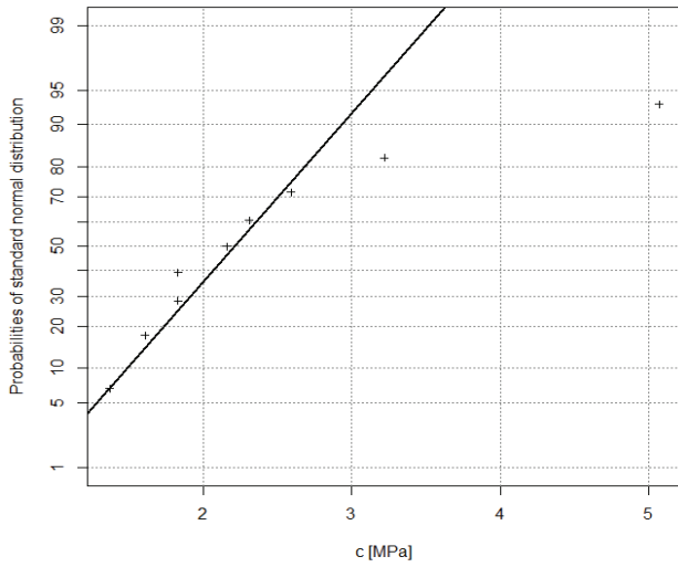
Kohäsion für tonreiches Haselgebirge
