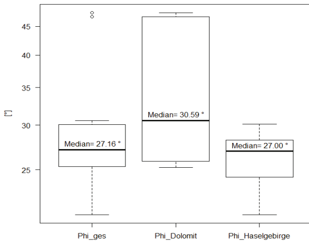
Reibungswinkel für Dolomit und Haselgebirge
