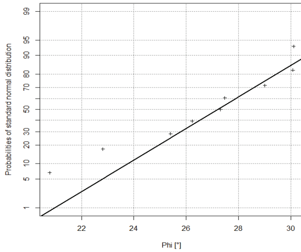
Reibungswinkel für tonreiches Haselgebirge
