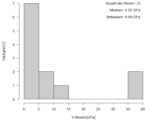
Verformungsmodul für Haselgebirge
