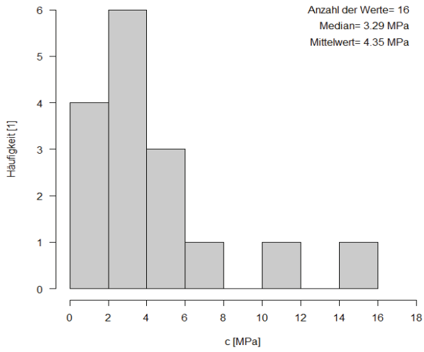
Kohäsion (c)
