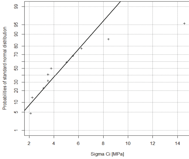
Sigma Ci für Haselgebirge
