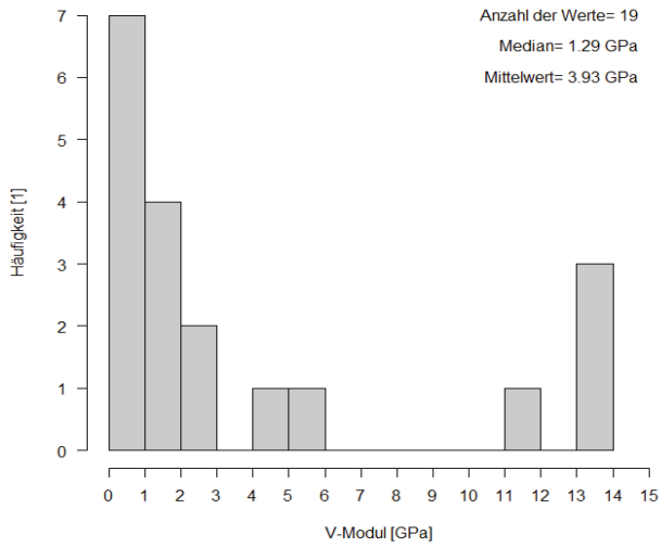
Verformungsmodul gesamt
