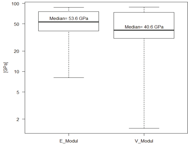
Elastizitäts- und Verformungsmodul für Dolomit
