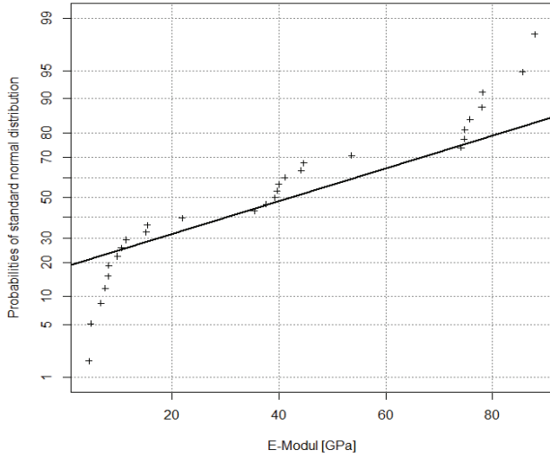
Elastizitätsmodul
