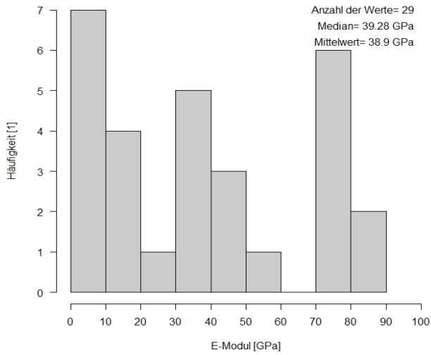
Elastizitätsmodul
