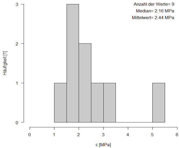
Kohäsion für tonreiches Haselgebirge
