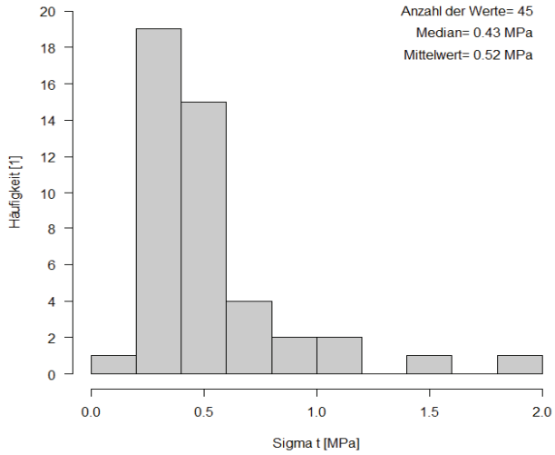
SPZ für Haselgebirge
