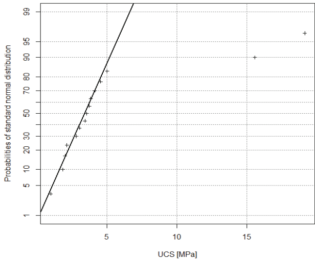
Einaxiale Druckfestigkeit für Haselgebirge
