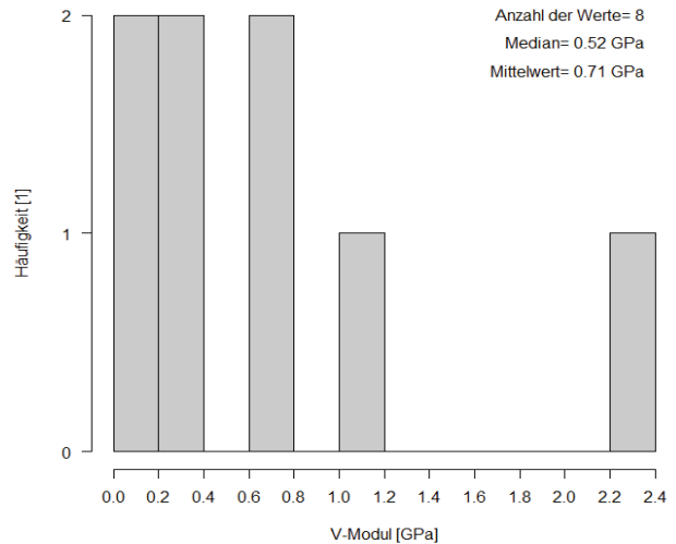
Verformungsmodul gesamt für tonreiches Haselgebirge
