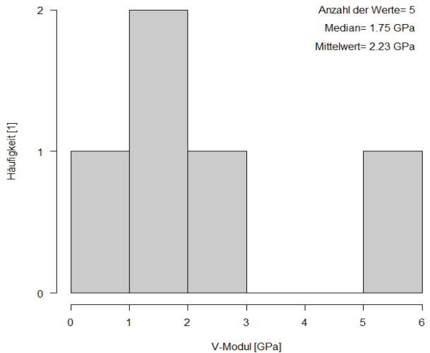
Verformungsmodul gesamt für gipsreiches Haselgebirge (ohne Ausreißer)
