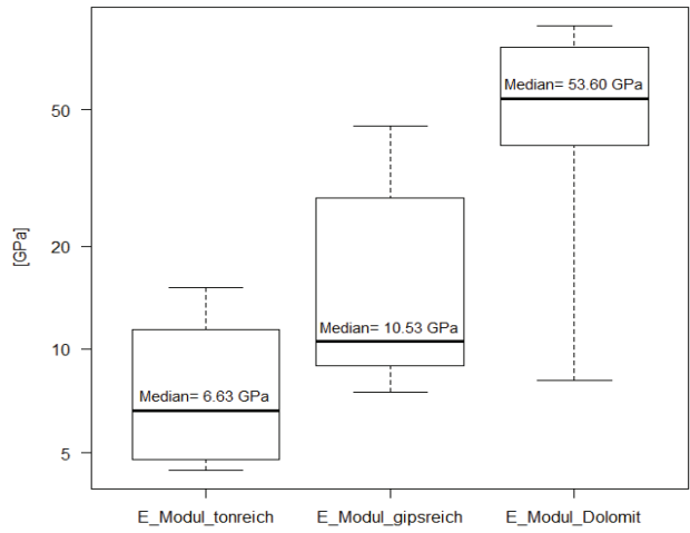
Elastizitätsmodul für ton-, gipsreiches Haselgebirge und Dolomit
