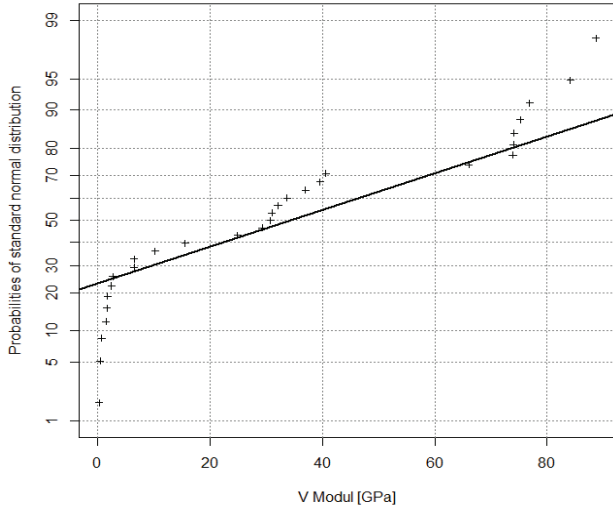
Verformungsmodul
