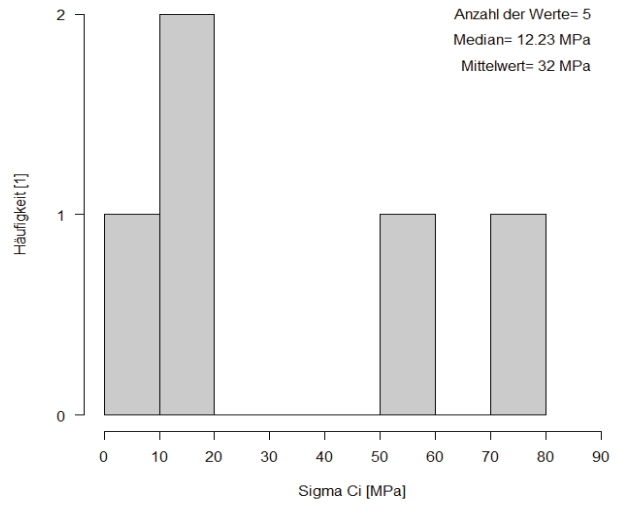
Sigma Ci für Dolomit
