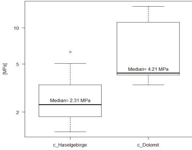
Kohäsion für Haselgebirge und Dolomit
