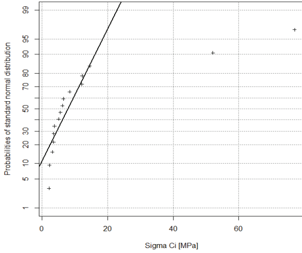
Sigma Ci
