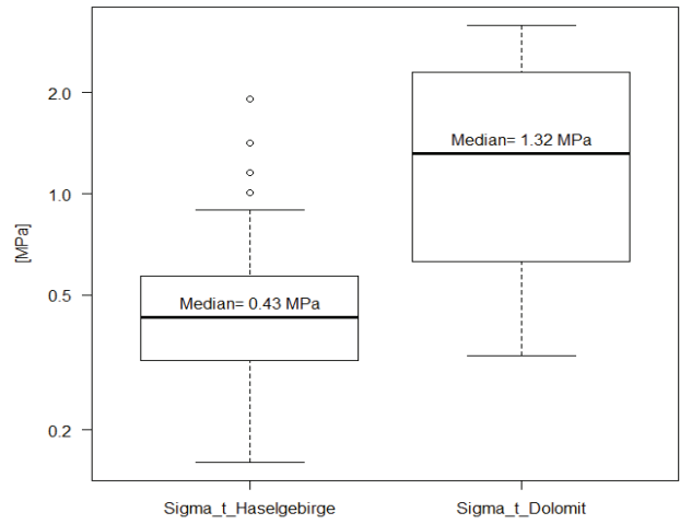
SPZ für Haselgebirge und Dolomit
