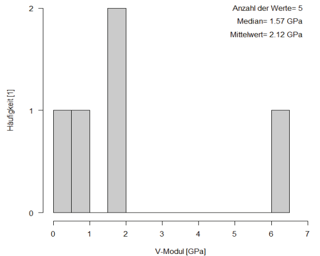
Verformungsmodul für tonreiches Haselgebirge
