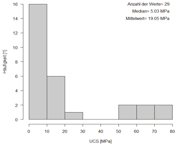
Einaxiale Druckfestigkeit (UCS)
