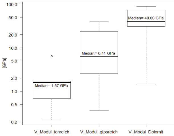
Verformungsmodul für ton-, gipsreiches Haselgebirge und Dolomit
