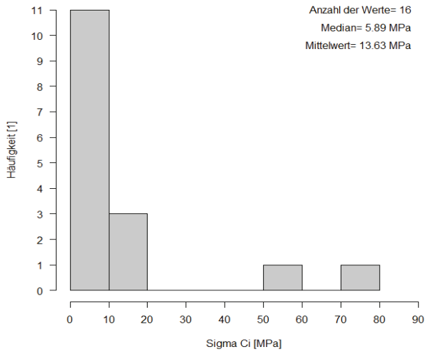
Sigma Ci
