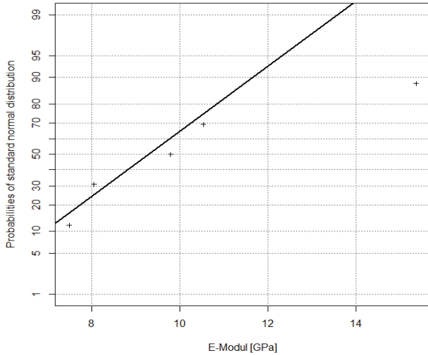
Elastizitätsmodul für gipsreiches Haselgebirge (ohne Ausreißer)
