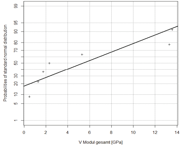
Verformungsmodul gesamt für gipsreiches Haselgebirge
