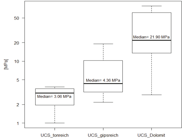
Einaxiale Druckfestigkeit für ton-, gipsreiches Haselgebirge und Dolomit
