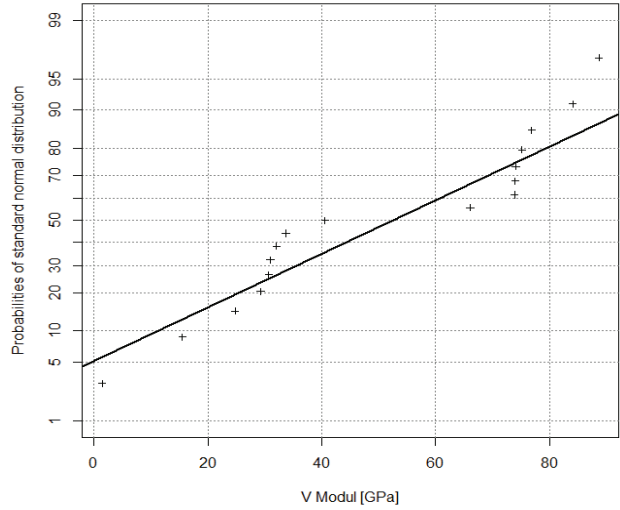
Verformungsmodul für Dolomit
