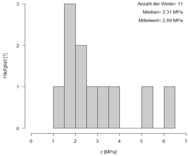
Kohäsion für Haselgebirge
