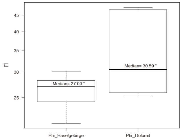
Reibungswinkel für Dolomit und Haselgebirge
