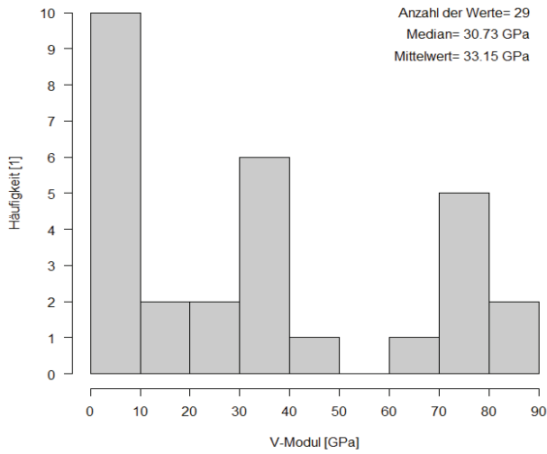
Verformungsmodul
