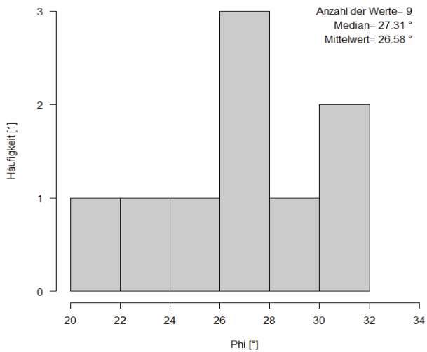
Reibungswinkel für tonreiches Haselgebirge
