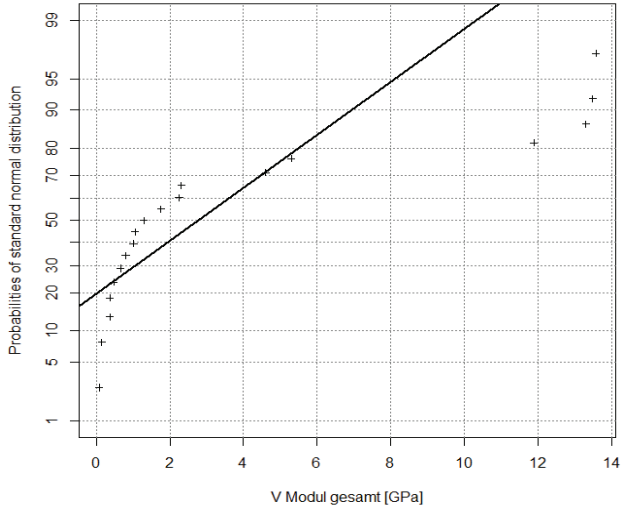
Verformungsmodul gesamt
