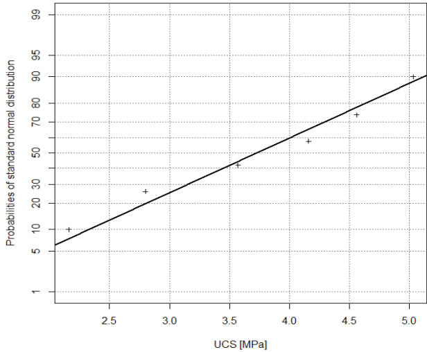
Einaxiale Druckfestigkeit für gipsreiches Haselgebirge (ohne Ausreißer)
