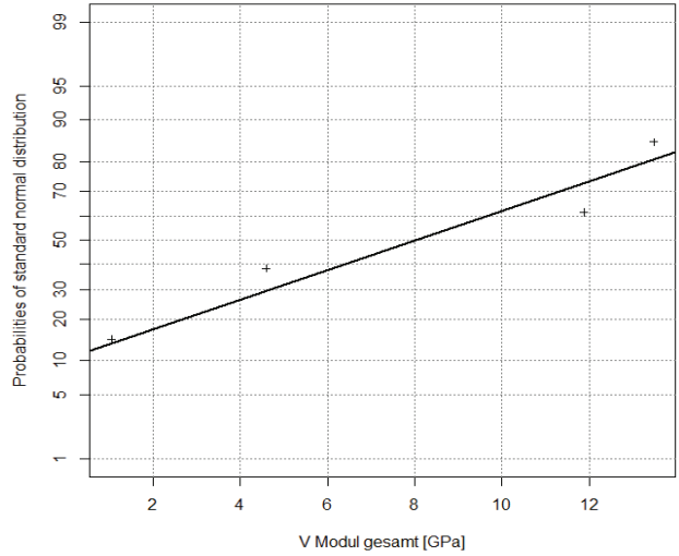
Verformungsmodul gesamt für Dolomit
