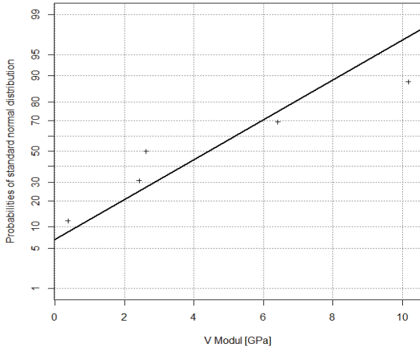
Verformungsmodul für gipsreiches Haselgebirge (ohne Ausreißer)
