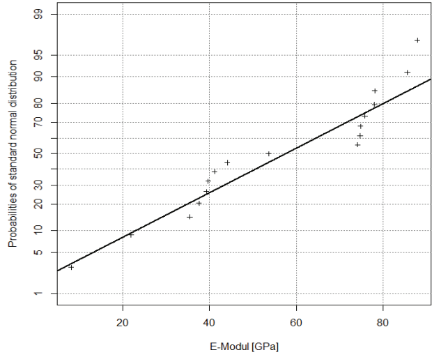
Elastizitätsmodul für Dolomit
