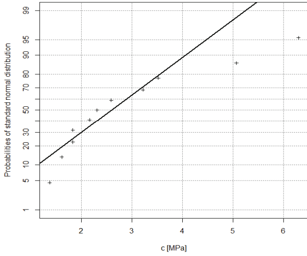
Kohäsion für Haselgebirge
