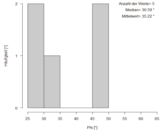
Reibungswinkel für Dolomit
