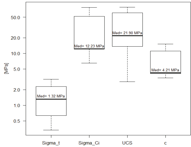
SPZ, Sigma Ci, UCS, c für Dolomit
